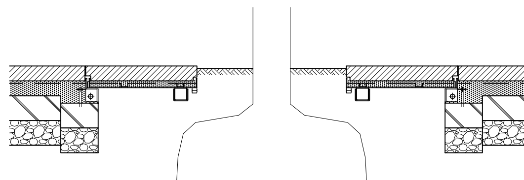
施工参考図
